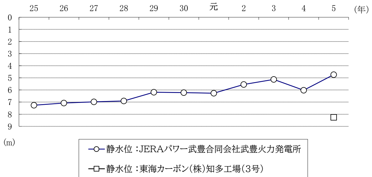
図5.1 地下水位経年変化
