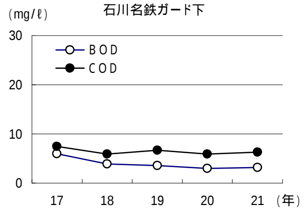
図 2 . 2 河川 B O D ・ C O D 経年変化
