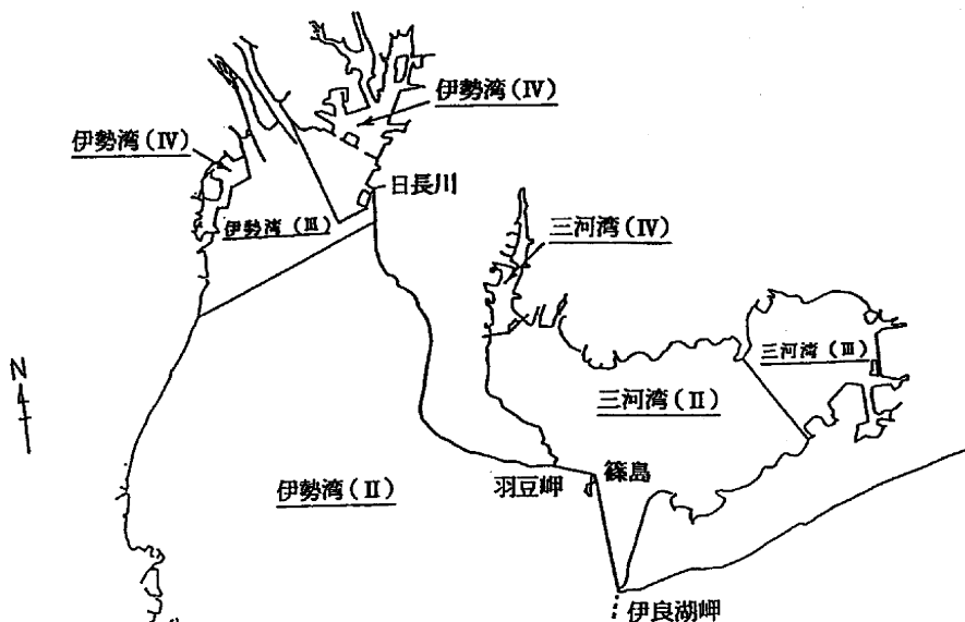
図2.5 伊勢湾・三河湾における全室素及び全りんに係る環境基準の水域類型指定
