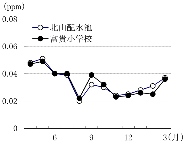
図１．１７ オキシダント(昼間)経月変化
