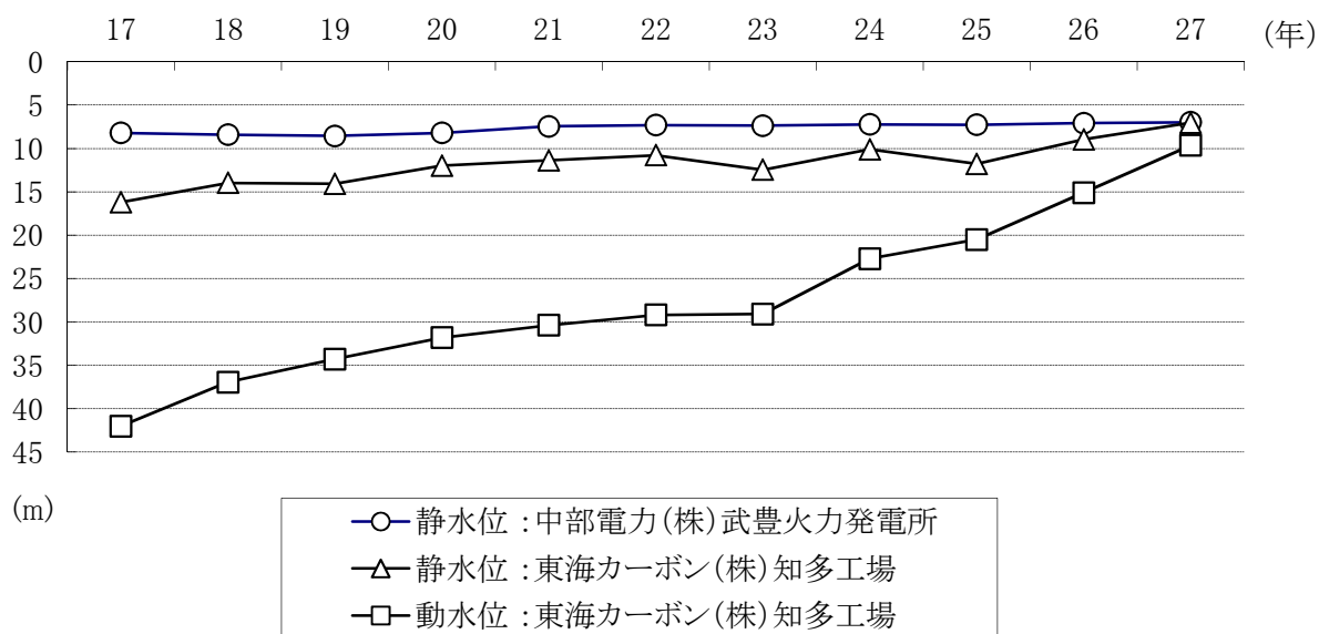
図5. 1 地下水位経年変化
