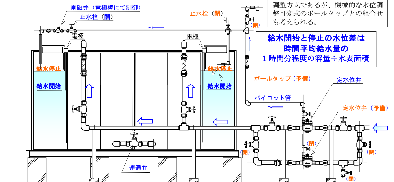
定水位弁周り配管要領図
