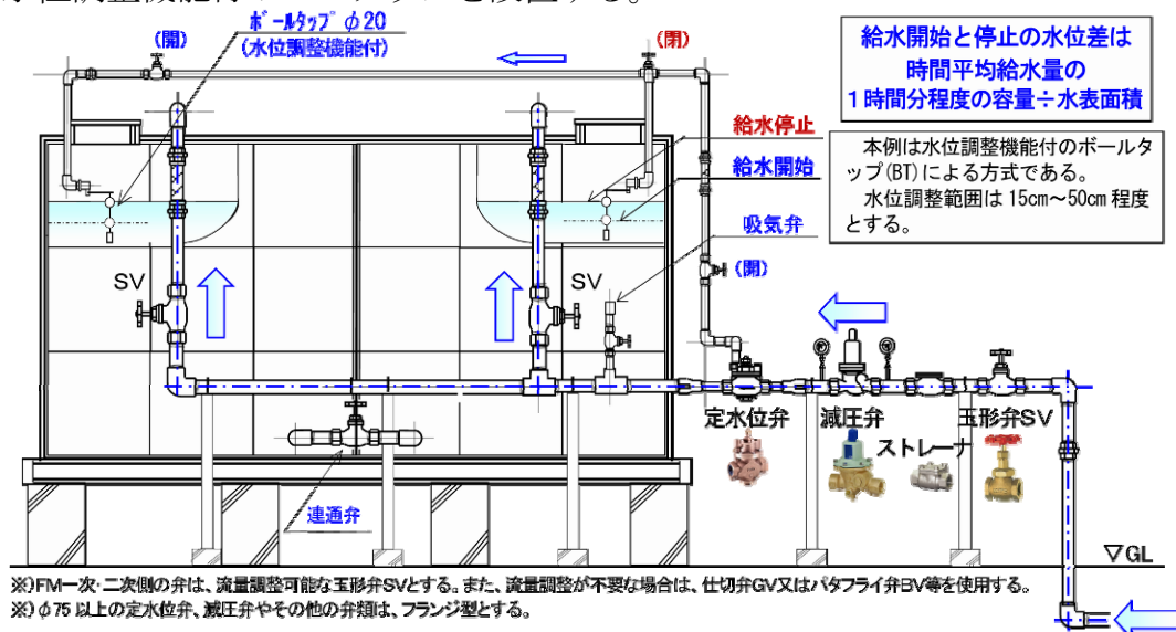
定水位弁及び減圧弁周りの配管要領図（その2）
