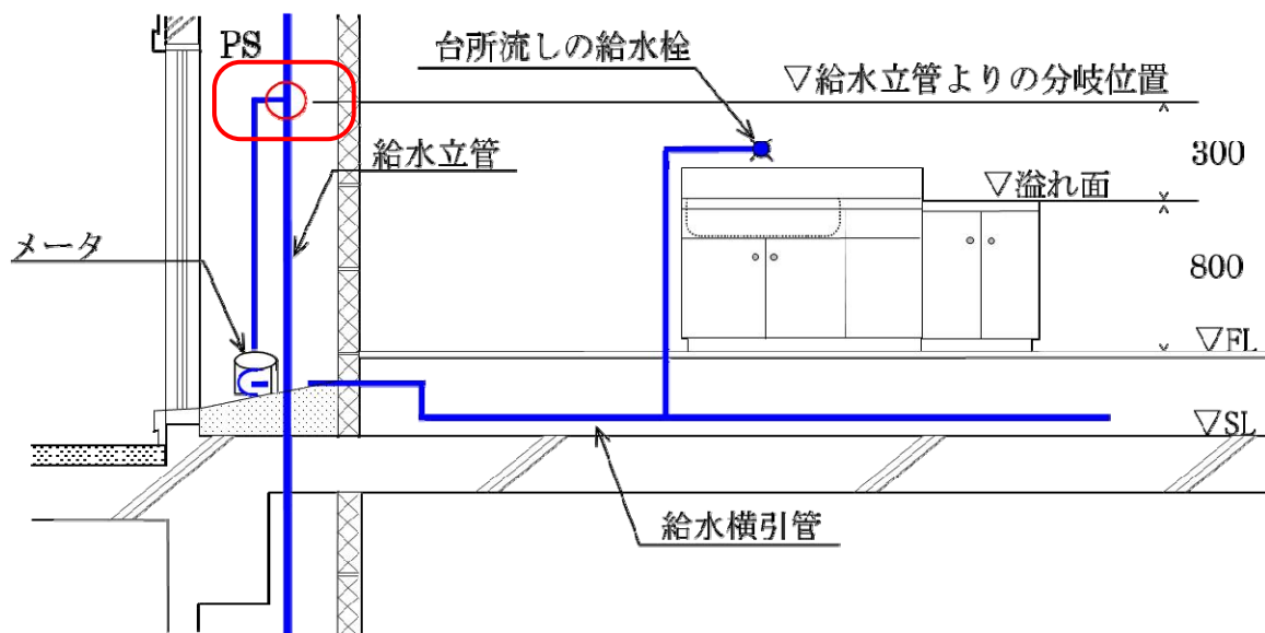
施工例－3
