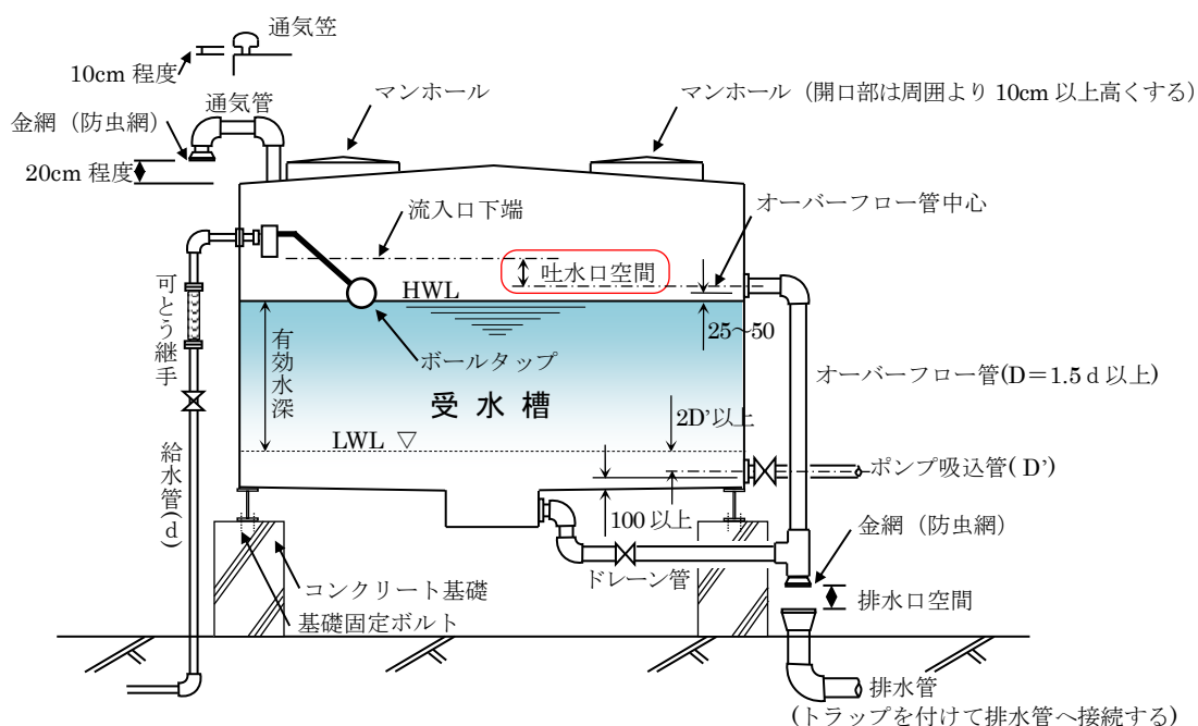
貯水槽における吐水口空間
