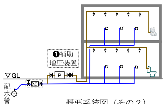
概要系統図 (その 2) (本町においては不可)
