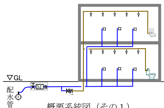
概要系統図 (その 1)
