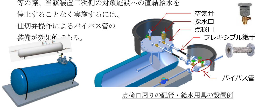
非常用貯水槽（例）
