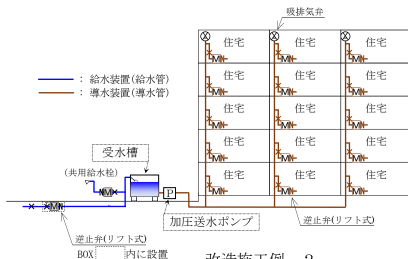
改造施工例-2
