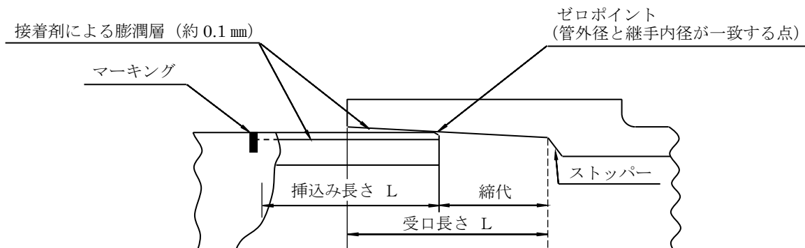
受口標準長さ
