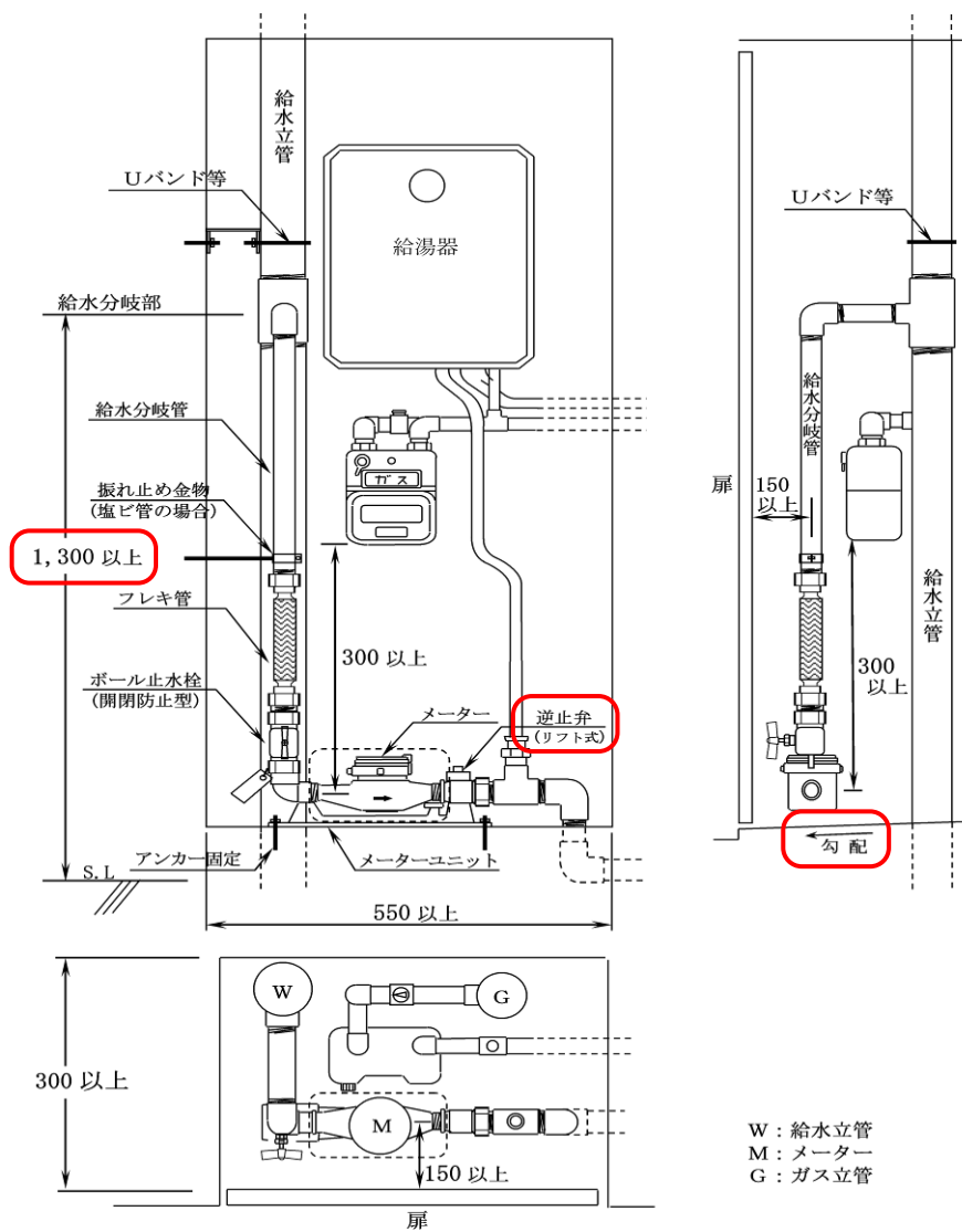
施工例－4
