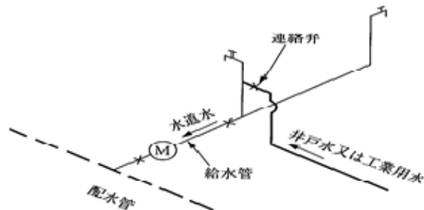
接続してはならない配管例
