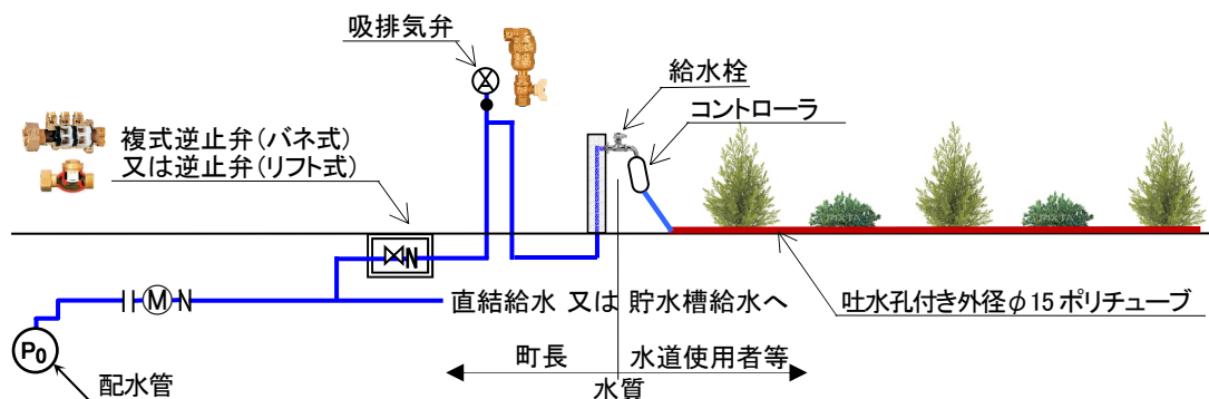
自動散水栓等周りの配管要領図 (例)
