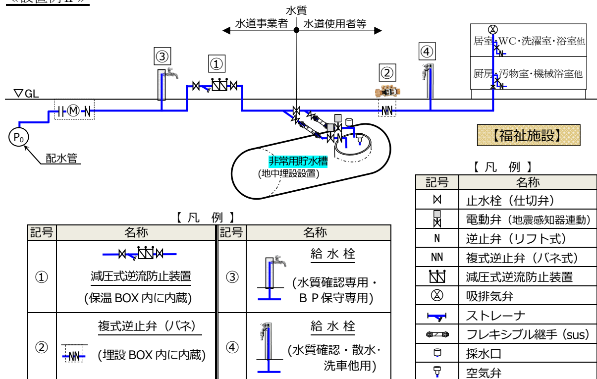
地中埋設型の非常用貯水槽の概略図－Ⅱ
