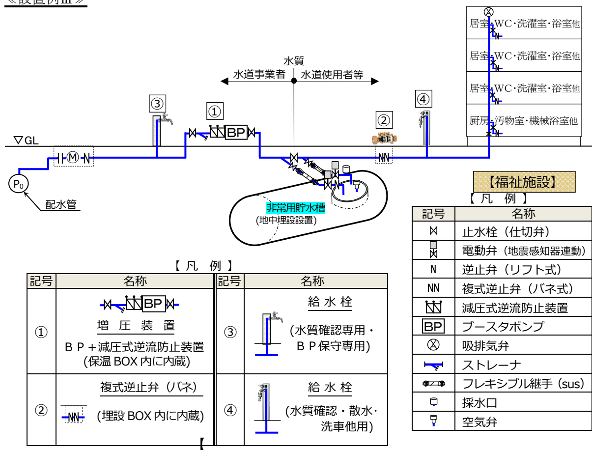
地中埋設型の非常用貯水槽の概略図－Ⅲ
