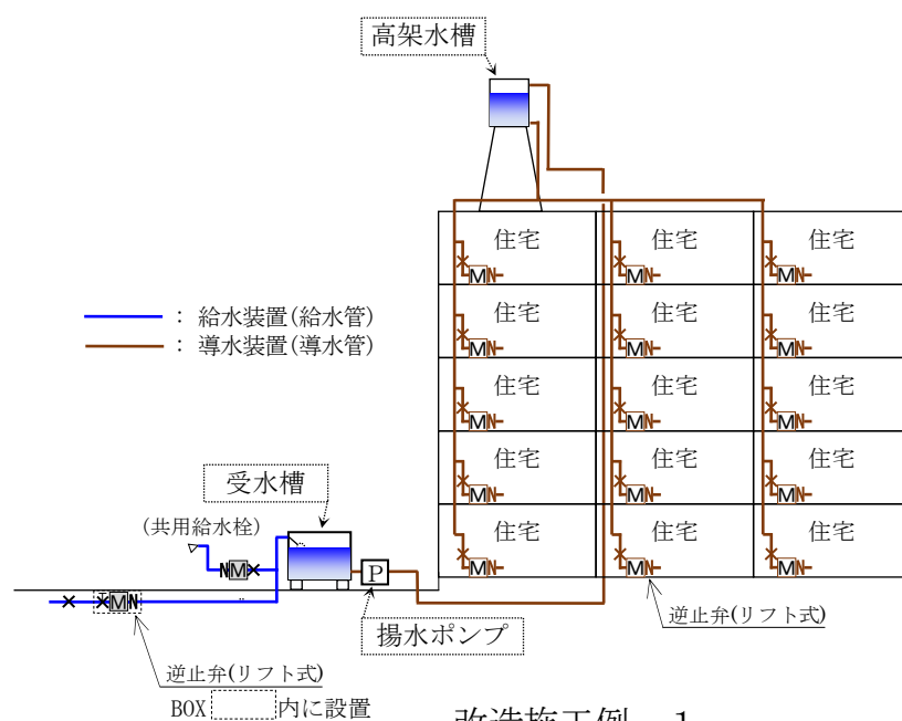
改造施工例-1
