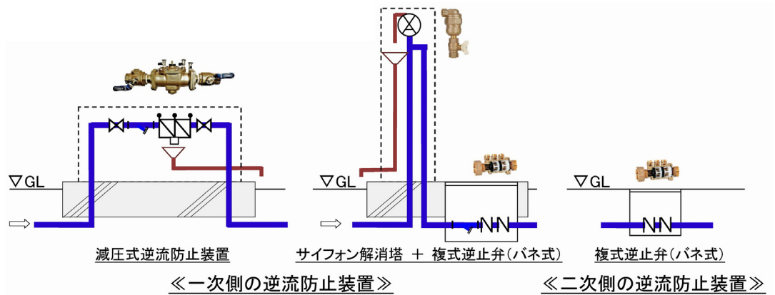
非常用貯水槽周りの逆流防止装置（例）
