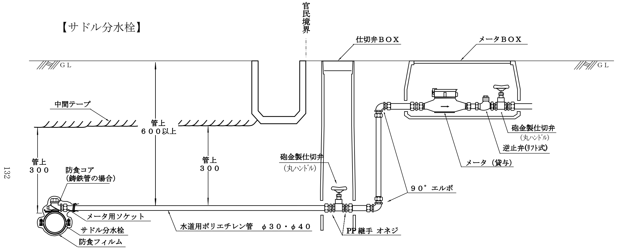
メータ口径 30・40mm 給水管取出し及びメータ設置標準図
