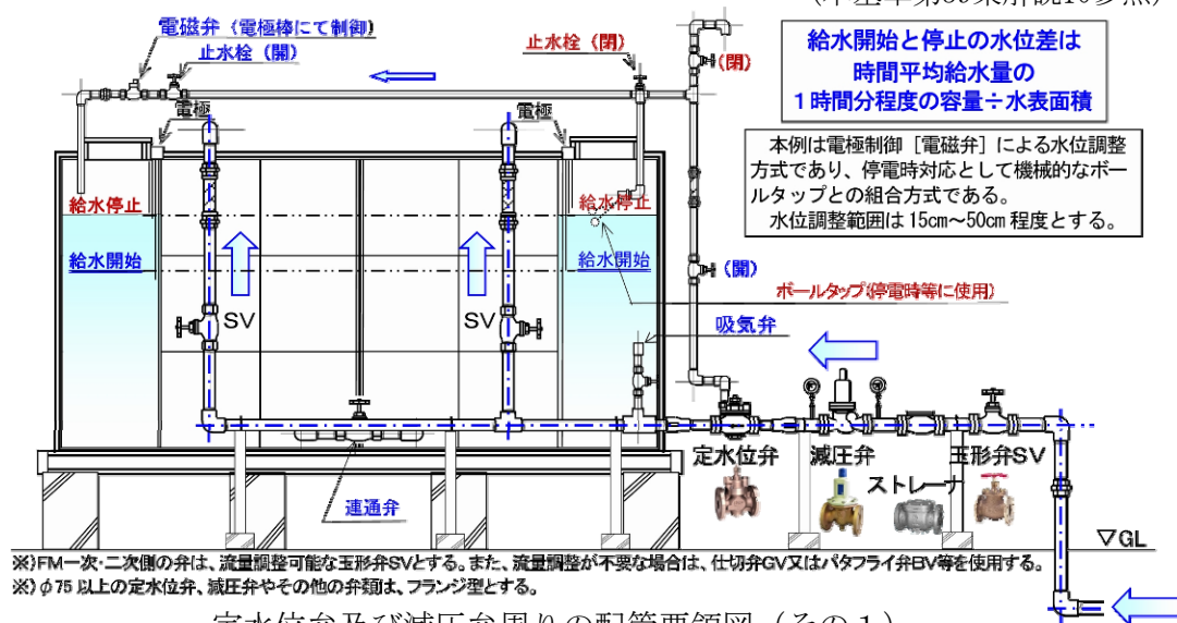
定水位弁及び減圧弁周りの配管要領図（その1）
