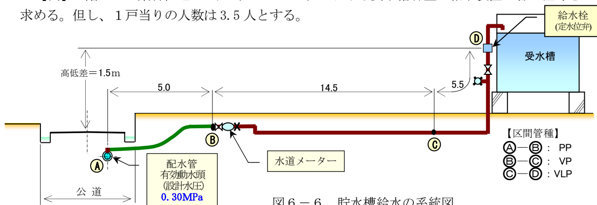
図6-6 貯水槽給水の系統図
