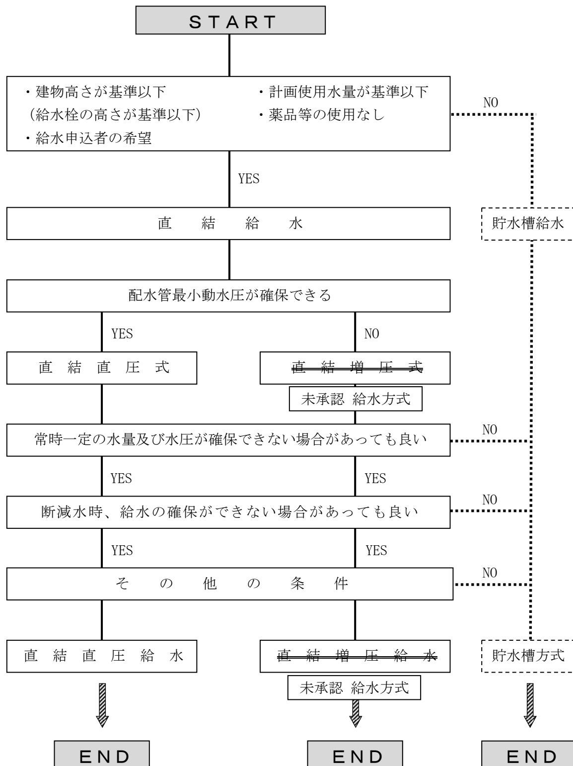
図1－2 給水形態の選定フロー（例）
