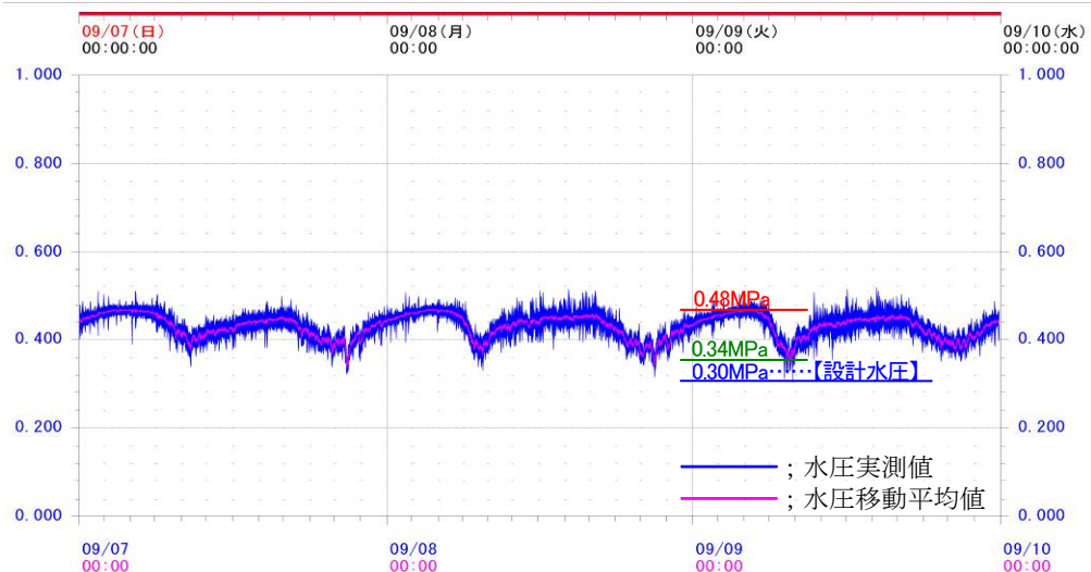
図6－7 水圧測定値（4秒間隔、3日間実測）
