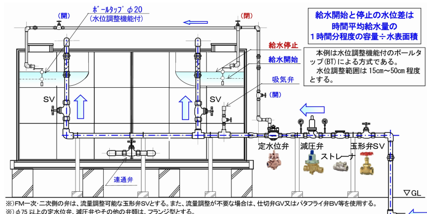
図 6－8 受水槽周り（一弁二槽型）の配管要領図
